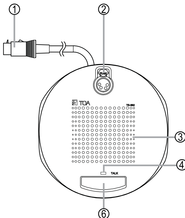
[TS-682-AS Top]
